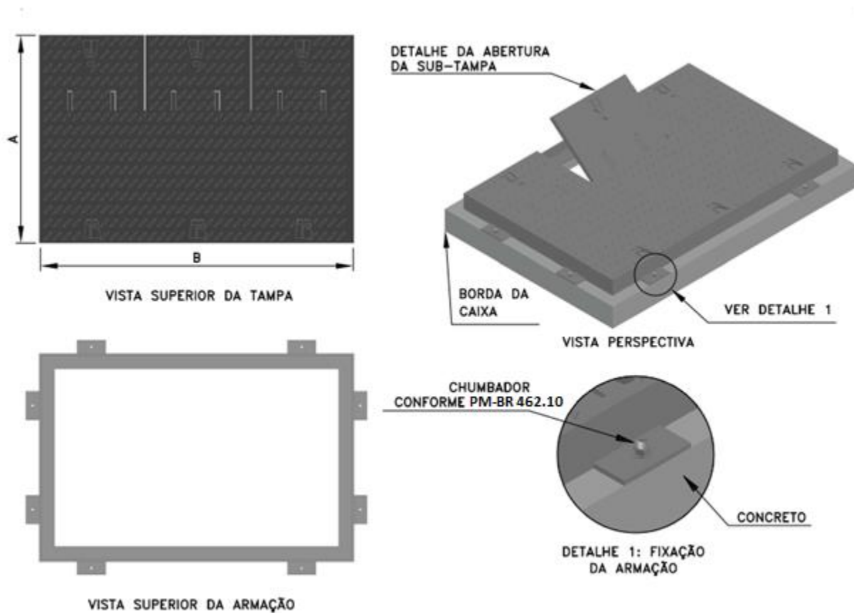
Figura 1 - Tampas de MT/BT
